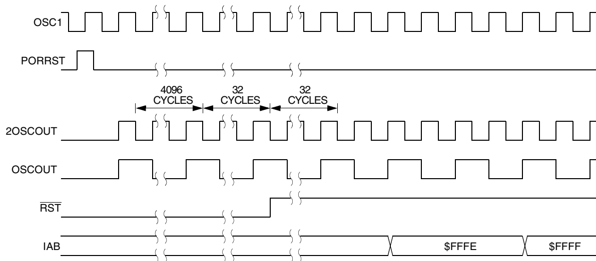
Figure 7-7. POR Recovery
